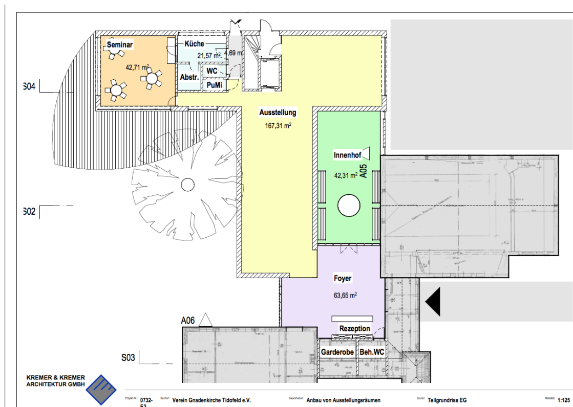
Abbildung 1: Entwurf Erdgeschoss
