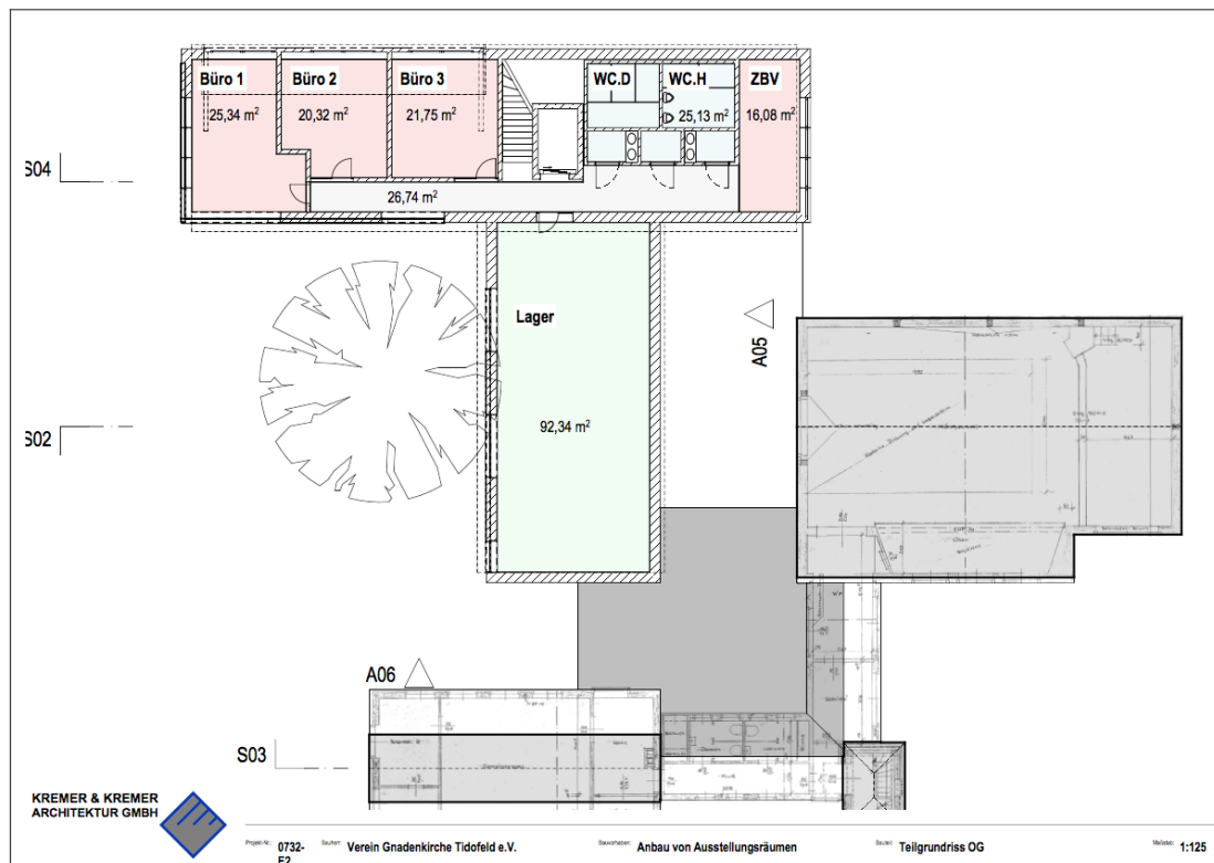
Abbildung 2: Entwurf Dachgeschoss
